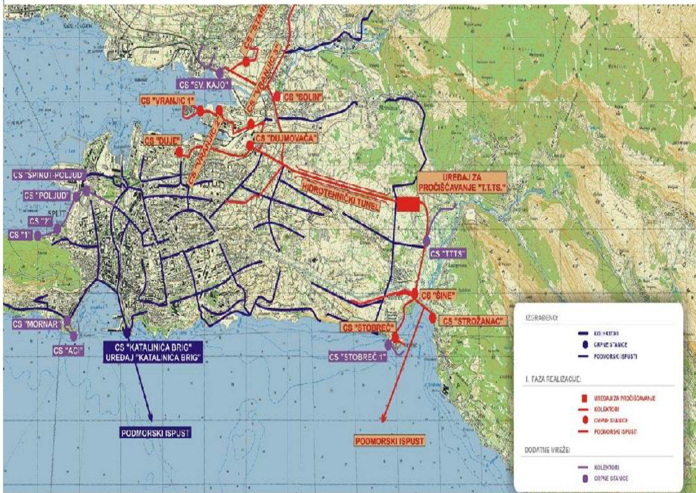
Slika 21: Isječak iz karte kanalizacijskog sustava Split – Solin (Izvor:URL12)
